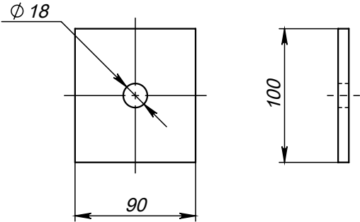
Поз.2 (Планка)
